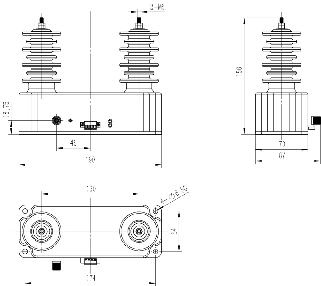
图 1 外形尺寸图
